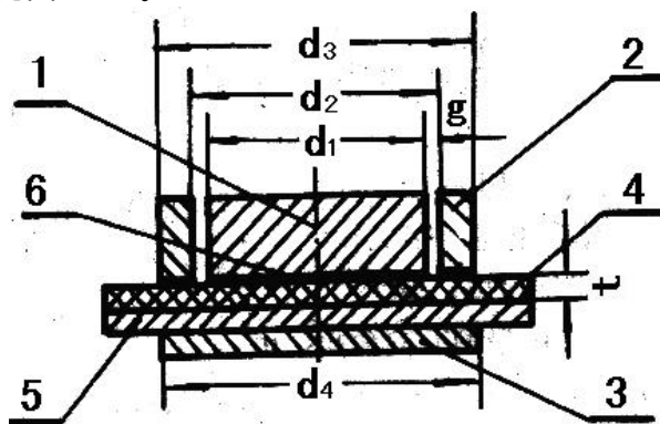
图 B.3.3 试件与电极配置
